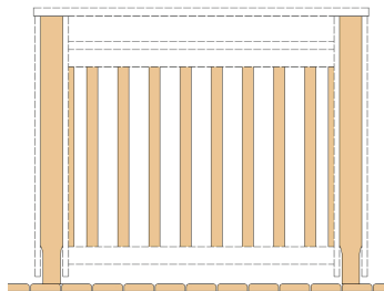
RÄCKE 34x45 STANDARD
