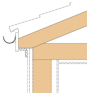
INKLÄDD INDRAGEN / KORT TAKFOT
