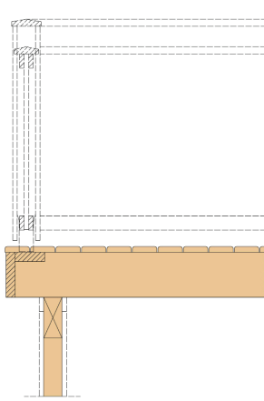
ÖPPEN BALKONG STANDARD
