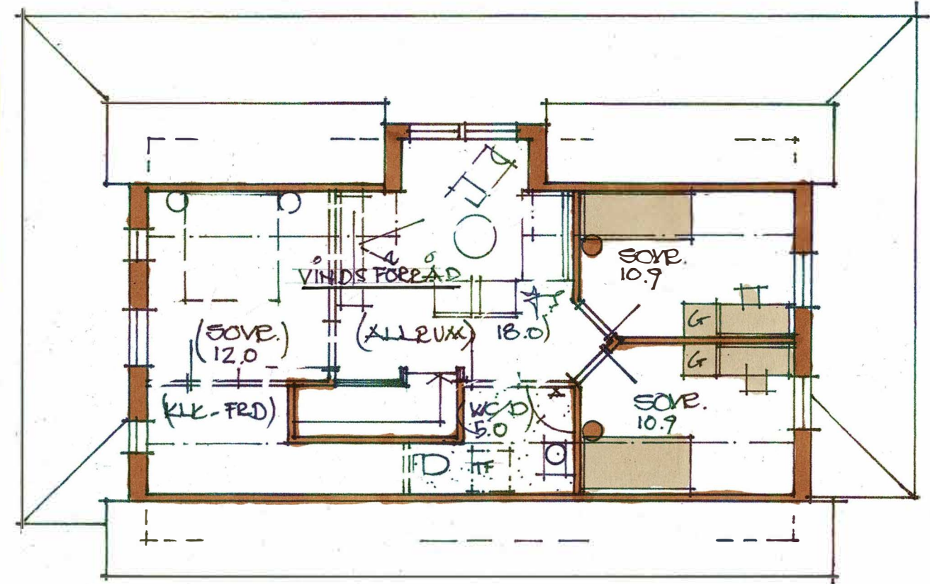
PLAN ITR. INV. AREA 67,2 m 2
