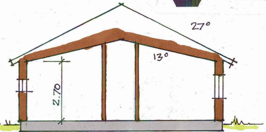
SEKTION a-a
