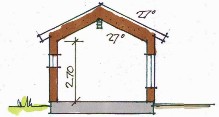
SEKTION b-b
