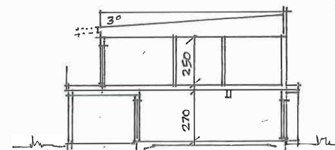
SEKTION a-a
